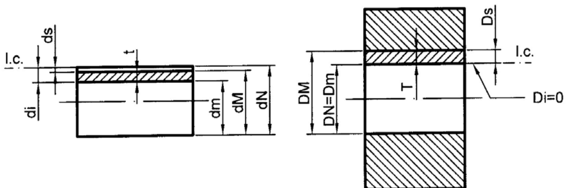
Figura 3. Croquis del eje y agujero con sus magnitudes características
